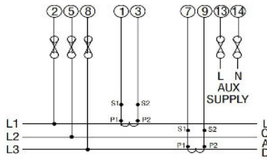
3PH - 3 Wire
