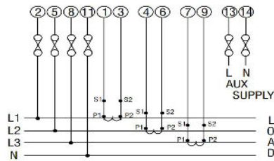
3PH - 4 Wire
