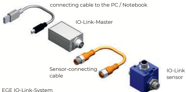
EGE IO-Link-System
